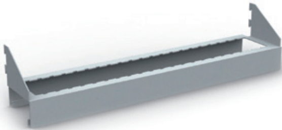
HALBFACHBODEN CNC | STATISCHE VARIANTE FÜR VERTIKALAUZUG AB 250 MM BREITE
